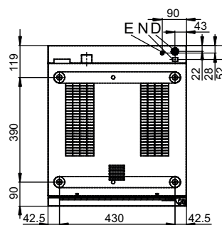
Positions de raccordement fond de l'appareil
