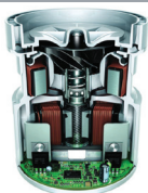
Moteur à impulsion numérique
