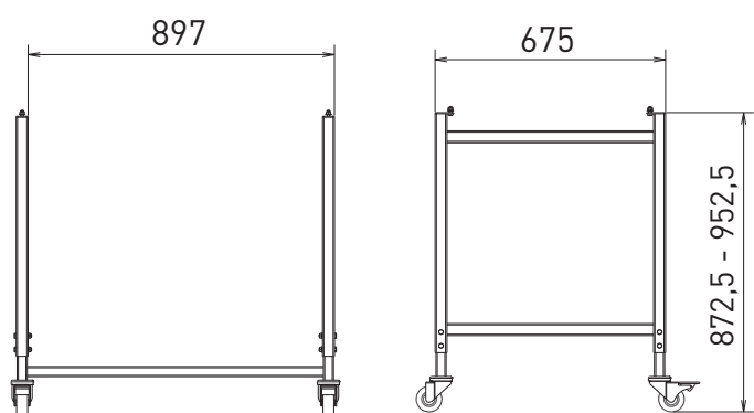
Dimensions socle simple (en mm)
