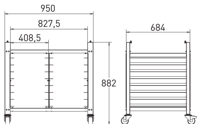
Dimensions socle avec rangement (en mm)
