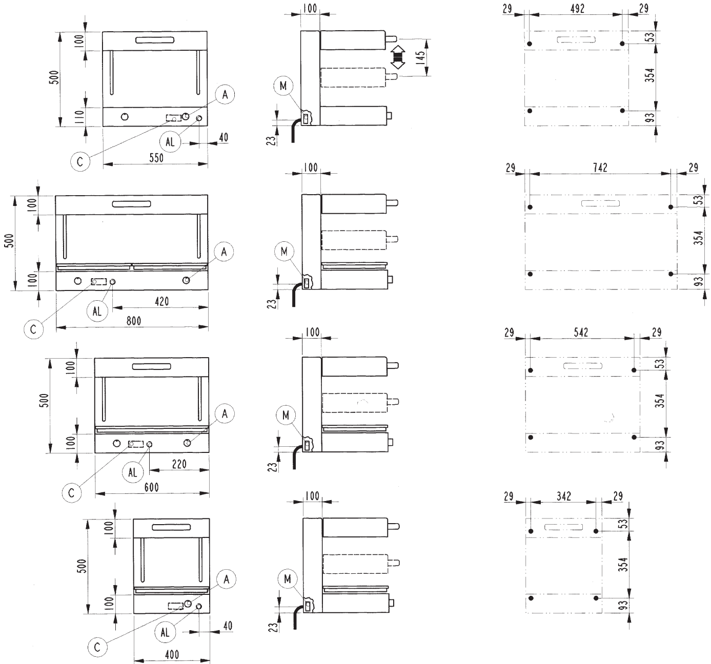
Schema di foratura parete in calcestruzzo per fissaggio staffe Schema für Betonwandbohrungen zur Befestigung der Wandhalterungen Diagram for drilling cement walls for the fastening of brackets Schéma de perçage de la paroi en béton pour fixer les étriers Esquema de perforación de la pared de hormigón para fijación soportes
