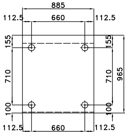
POSIZIONE PIEDINI
