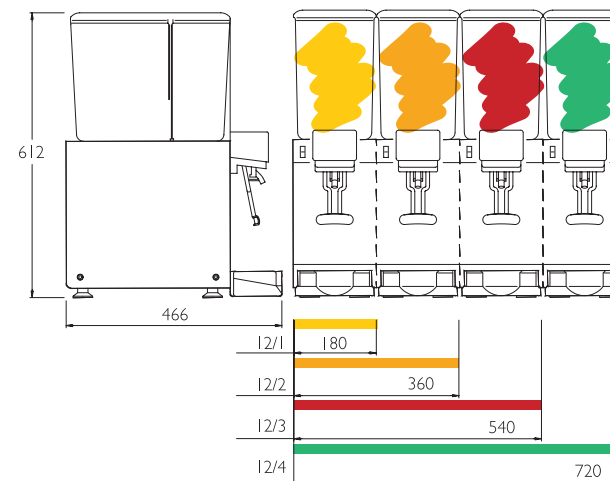
Modelli 12/1, 12/2, 12/3 e 12/4
