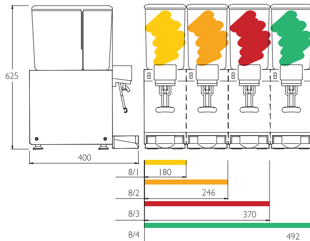
Modelli 8/1, 8/2, 8/3 e 8/4
