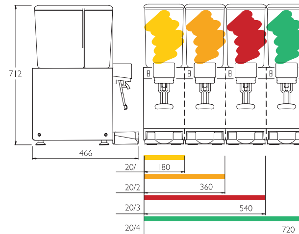
Modelli 20/1, 20/2, 20/3 e 20/4
