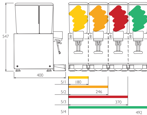
Modelli 5/1, 5/2, 5/3 e 5/4
